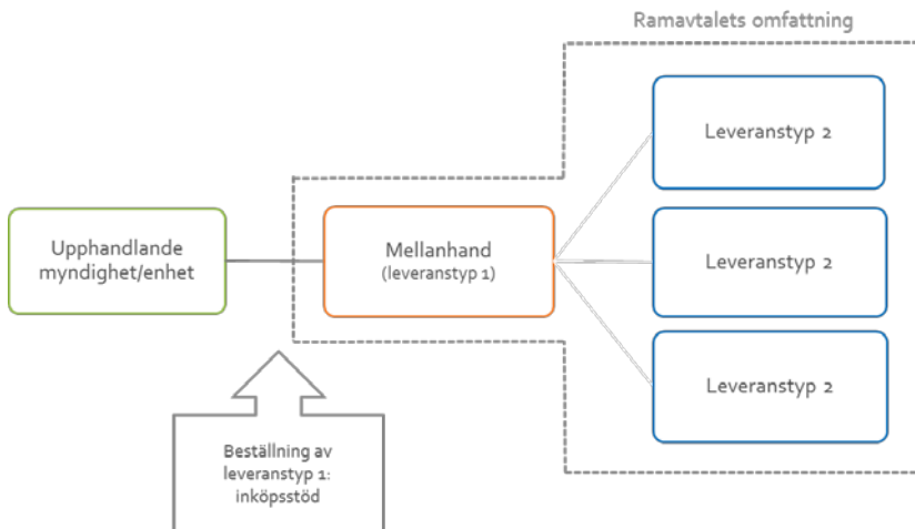
Figur 11: Underleverantörlösningen (avrop 1)
