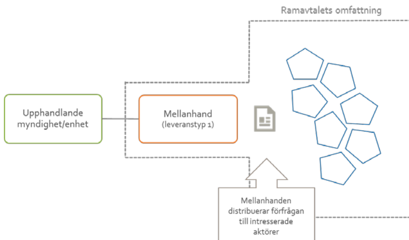
Figur 12: Underleverantörlösningen (konkurrensutsättning)
