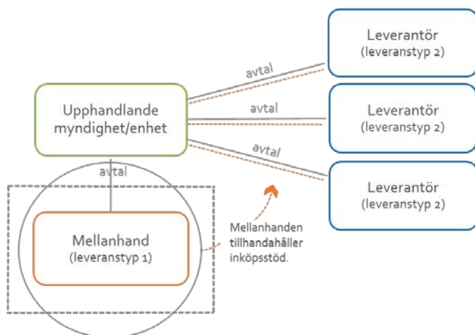
Figur 18: Mäklarlösningen (upphandling)
