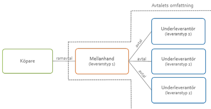
Figur 2: Underleverantörlösningen (definition)
